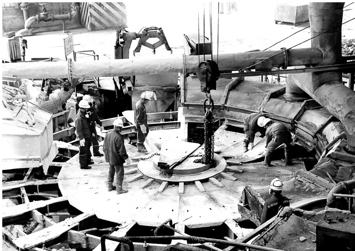
金隆铜业公司正在对阳极板生产的关键设备圆盘浇铸系统进行维修(如图)。上半年,该公司利用设备全面检修的机会,对圆盘浇铸机进行投产以来的第一次检修,以促进未来生产。七月份,该公司阳极板产量超过五万吨,创造了投产以来单月产量最高的历史纪录。 章 庆 摄
