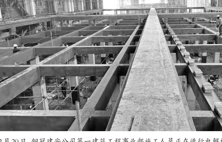
12月20日,铜冠建安公司第一建筑工程事业部施工人员进行电解槽支架施工。由铜冠建安公司第一建筑工程事业部承建的铜基新材料项目电解车间施工日前取得新进展,其中电解工段顺利通过GH轴14-25线、32-53线电解槽支架防腐蚀,提前完成工序交接工作。
