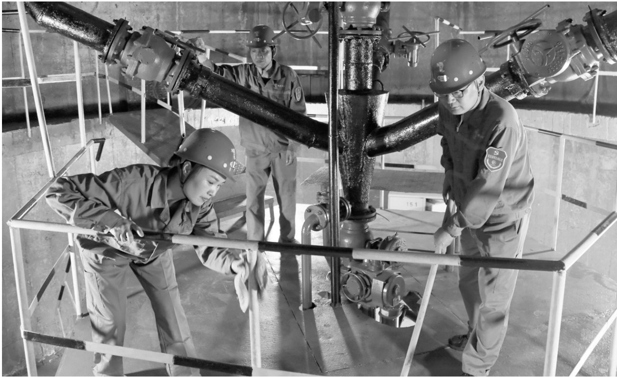
连日来,安庆铜矿工程工区扎实推进5S精益管理“设备见本色”活动,集中精干突击力量,对该区充填站进行全面整治,先后对三个搅拌桶及所有楼梯栏杆进行清污、除锈、刷漆,对充填水管、风管、送砂管按规定要求刷涂标准色漆,共刷涂管道200余米,清理电机灰渍、油污20台套,真正使站内各类设备、设施见了“本色”。图为当班人员正在对整治后的设备进行日常清扫维护。 程海滨 摄
