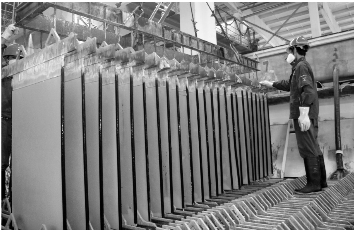
10月份,铜冠池州公司锌产品产量突破至12967吨,创月度产量历史新高,其中锌合金产量达到4750吨,持续保持产量高位运行。图为员工装出槽作业。张军 摄
