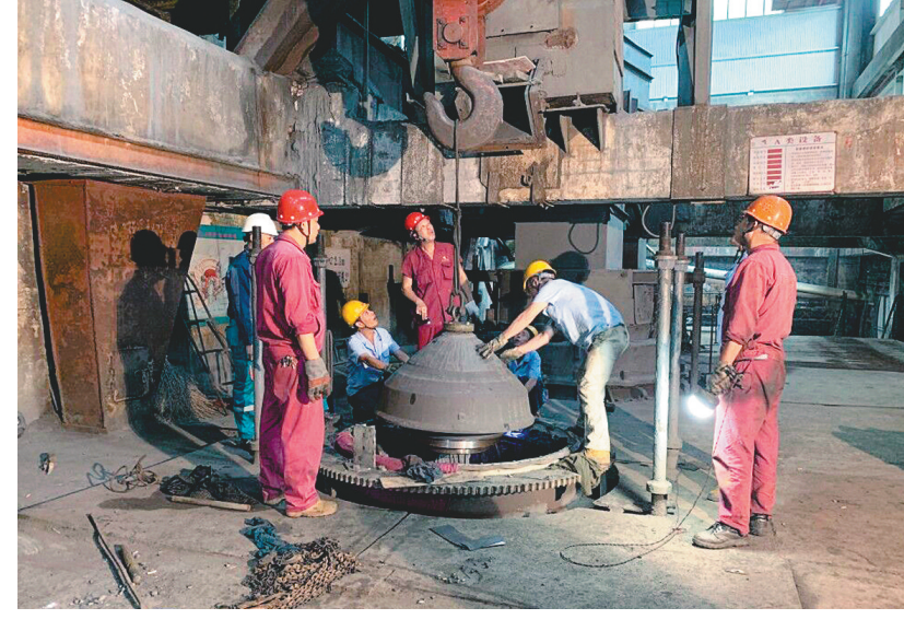
日前,天马山矿业公司选矿车间圆锥破碎机HP300主轴偏心铜套出现抱死现象,导致设备无法运转。车间积极组织人员进行抢修,在厂家技术人员的指导下,首次对设备传动部分进行了拆除检修,目前设备进入安装调试阶段。图为维修人员吊装破碎机动锥。 王刚强 朱艳摄
