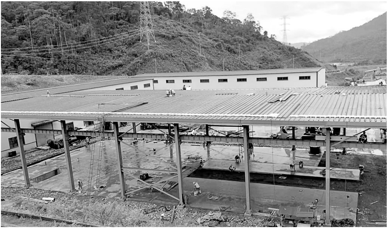
铜冠建安厄瓜多尔分公司员工利用下雨间隙进行施工(如图)。由铜冠建安厄瓜多尔分公司承建的米拉多铜矿铜焊车间工程已进入收官阶段,目前屋面打瓦、行车安装、地面混凝土浇筑等全面展开,分公司克服多雨天气影响,全力确保提前完成该工程施工任务。
