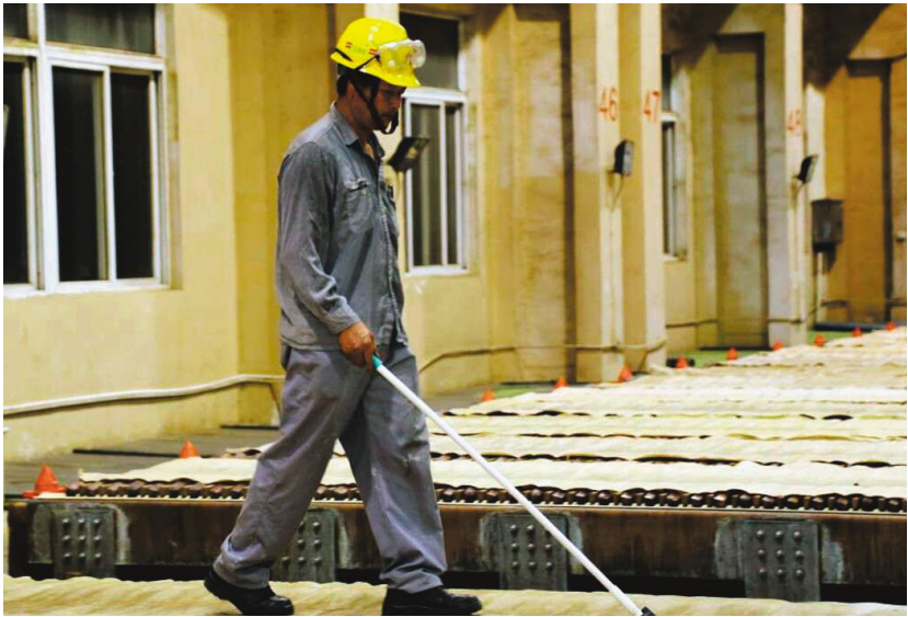
金冠铜业公司电解车间员工在槽面检查短路。
